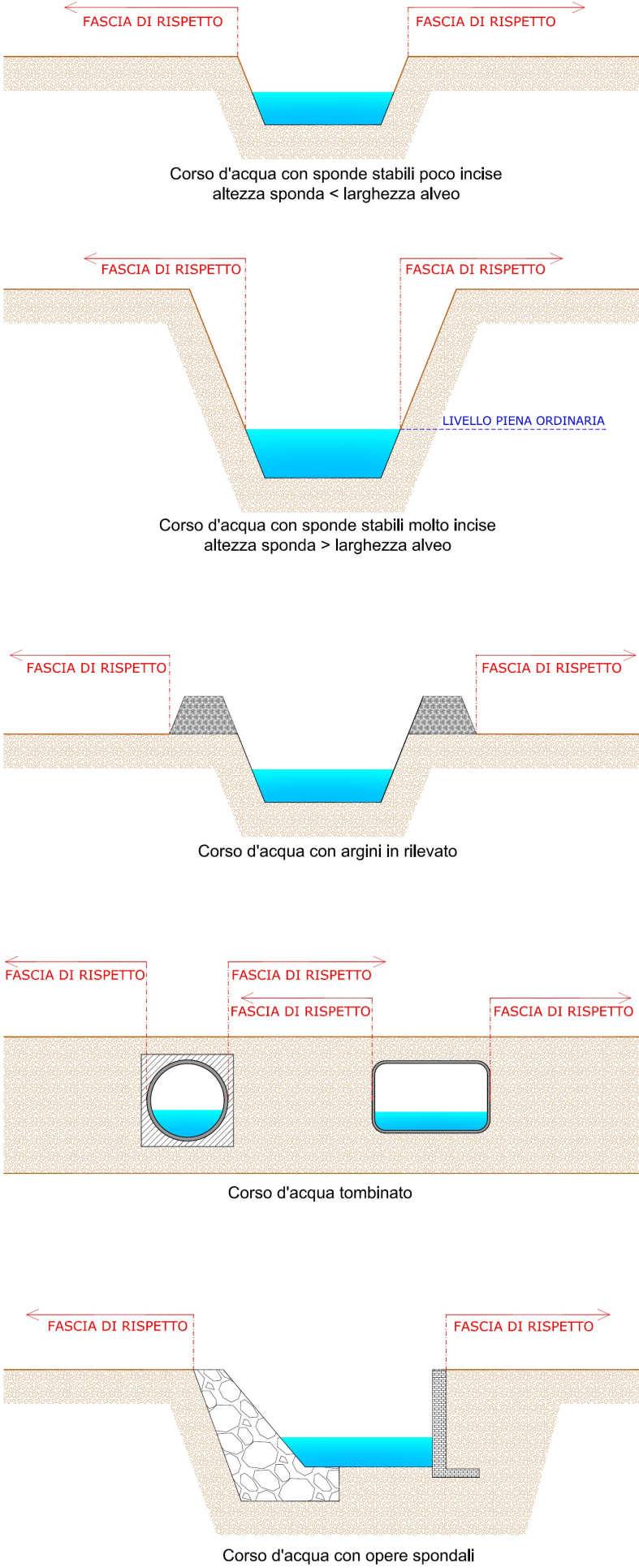
ESEMPI SCHEMATICI PER LA CORRETTA DELIMITAZIONE DELLE FASCE DI RISPETTO IDRAULICO DA APPLICARE IN SITO
